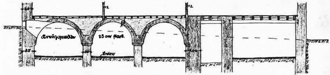
Сchnitt - А-Б.
